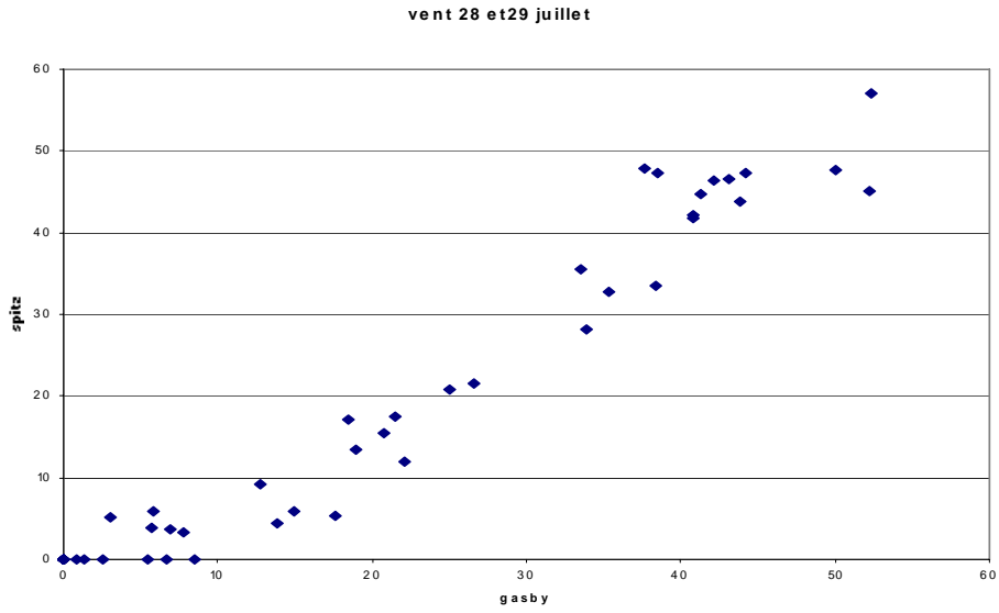
Graphique 2 : Variation du vent à Gásby et à la Base les 28 et 29 juillet (temps couvert)
