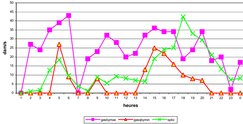
graphique 4 : Comparaison de la vitesse du vent entre les deux stations le 20 juillet
