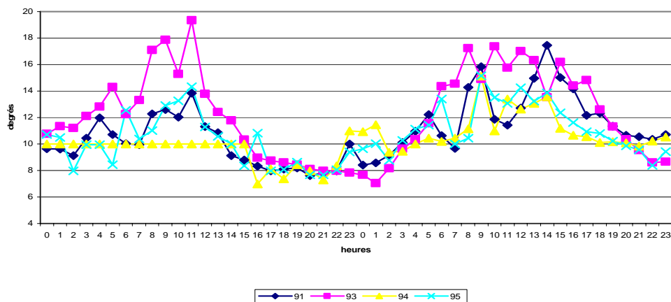
Graphique 1 : Variation des températures horaires les 19 et 20 juillet en 4 stations
