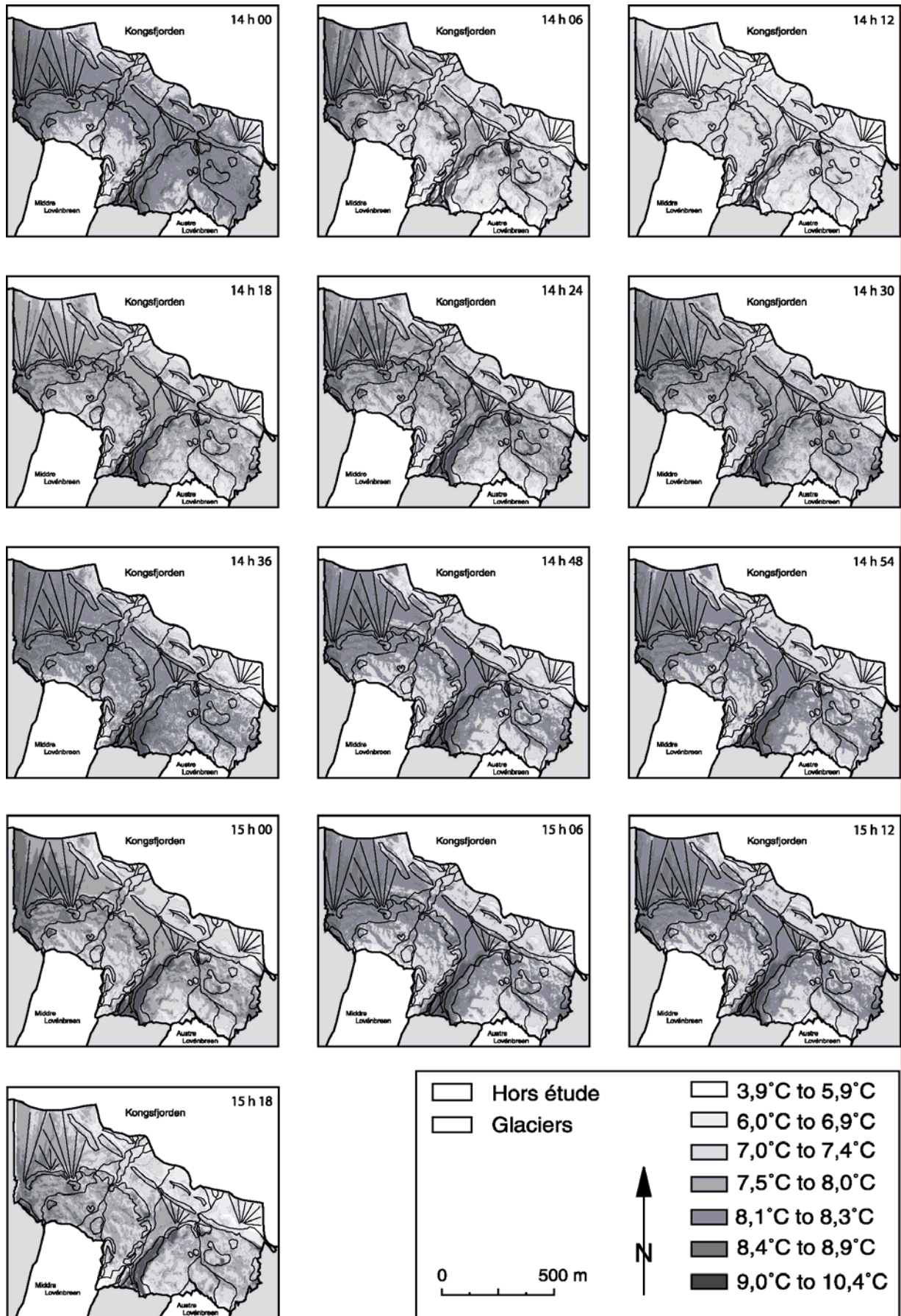
Figure 2 : Températures à intervalle de 6 minutes de 14 h 00 à 15 h 18 le 20 juillet 1999
