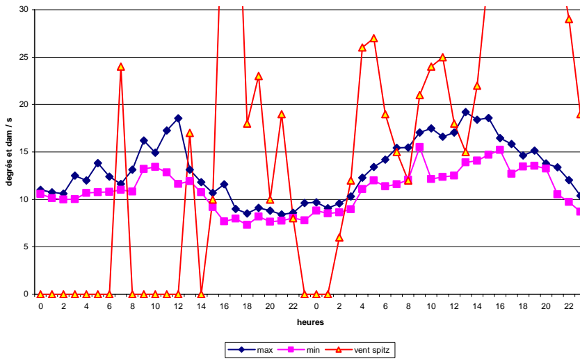
graphique 5 : Comparaison de la variation du vent et de la température les 19-20 juillet à la Base
