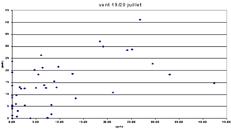
Graphique 3 : Variation du vent à Gåsby et à la Base les 19 et 20 juillet (temps ensoleillé).
