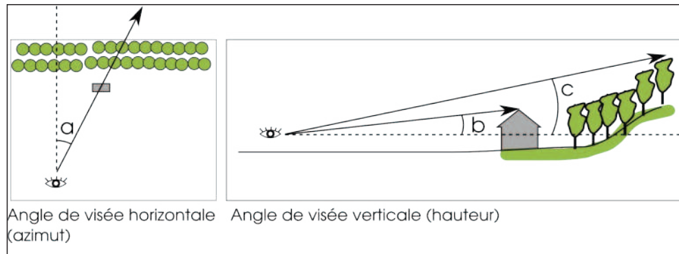
Figure 2.8. Les calculs des angles de visée horizontale et verticale à la base de la modélisation des visibilitées
